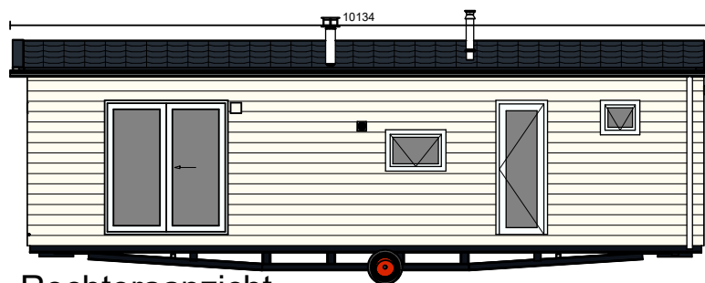
Rechteraanzicht
