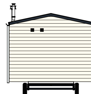
Achteraanzicht
